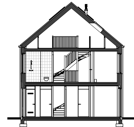
DOORSNEDE B
