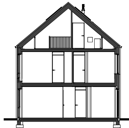
DOORSNEDE A
