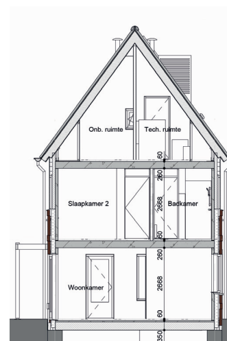
Doorsnede C2
