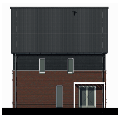
Zijgevel C2
