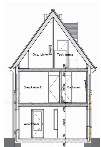
Doorsnede C1
