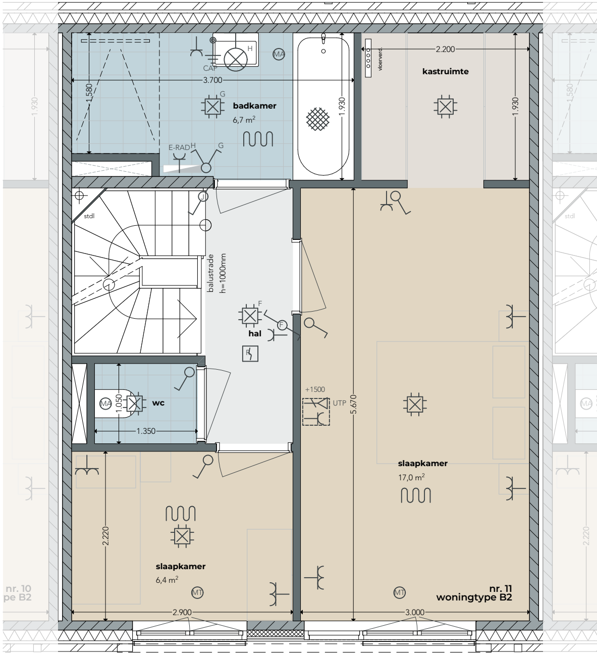
1e verdieping schaal 1:50
