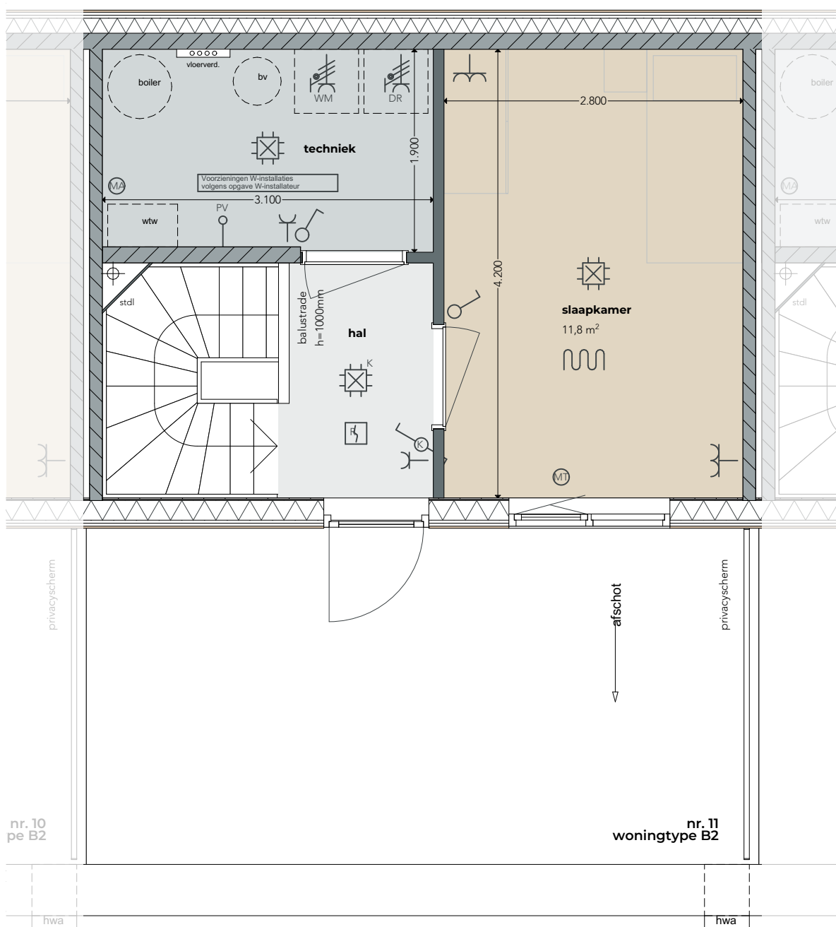
3e verdieping schaal 1:50
