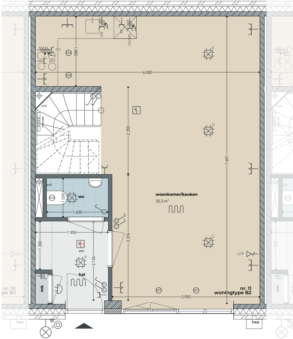
Begane grond schaal 1:50
