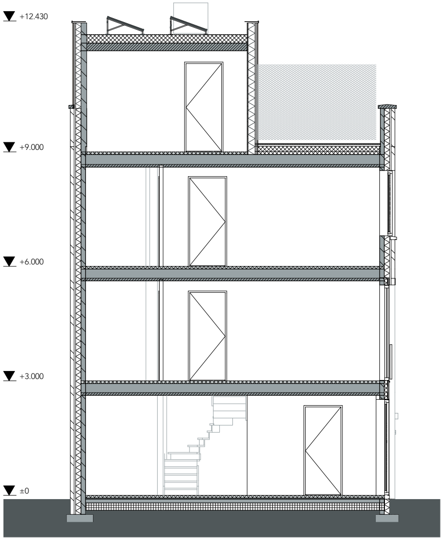
doorsnede schaal 1:100
