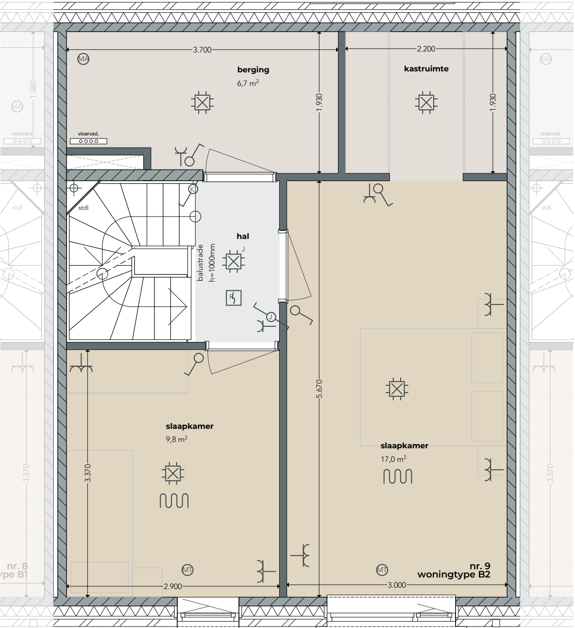
2e verdieping schaal 1:50
