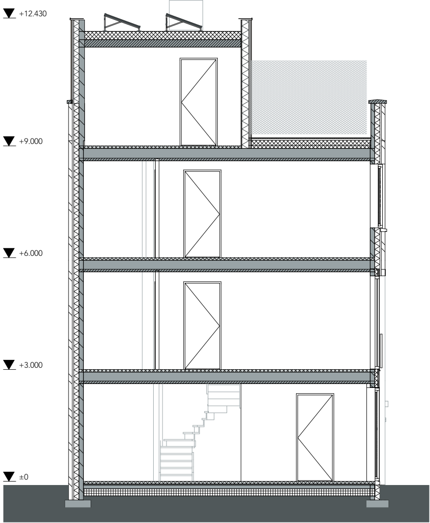
doorsnede schaal 1:100
