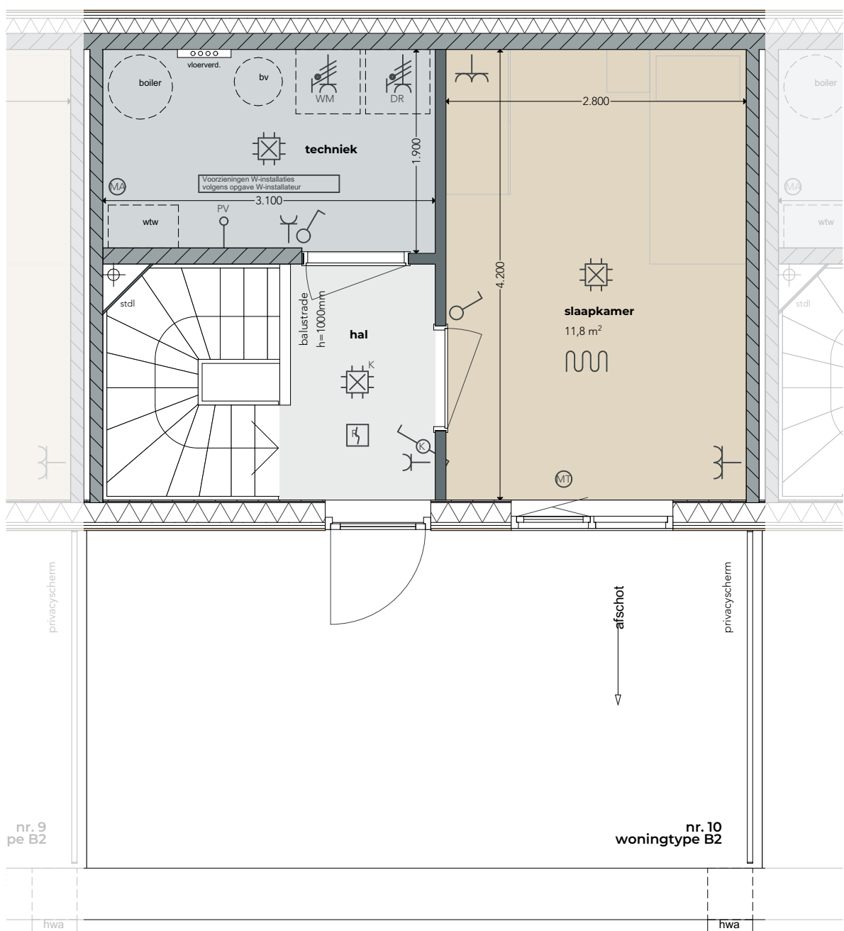
3e verdieping schaal 1:50
