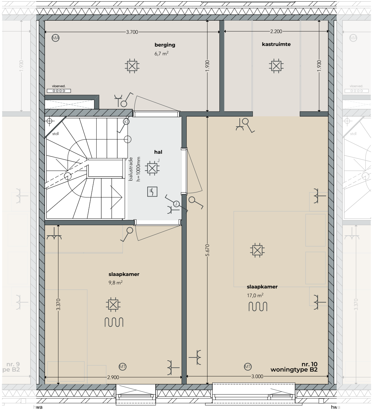
2e verdieping schaal 1:50
