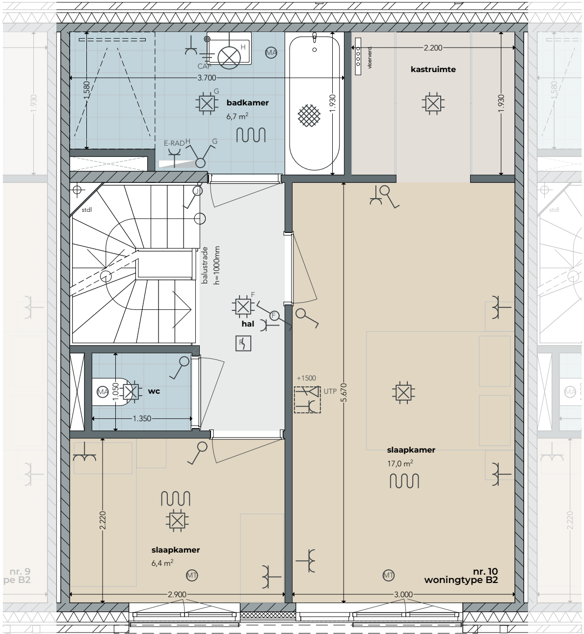
1e verdieping schaal 1:50
