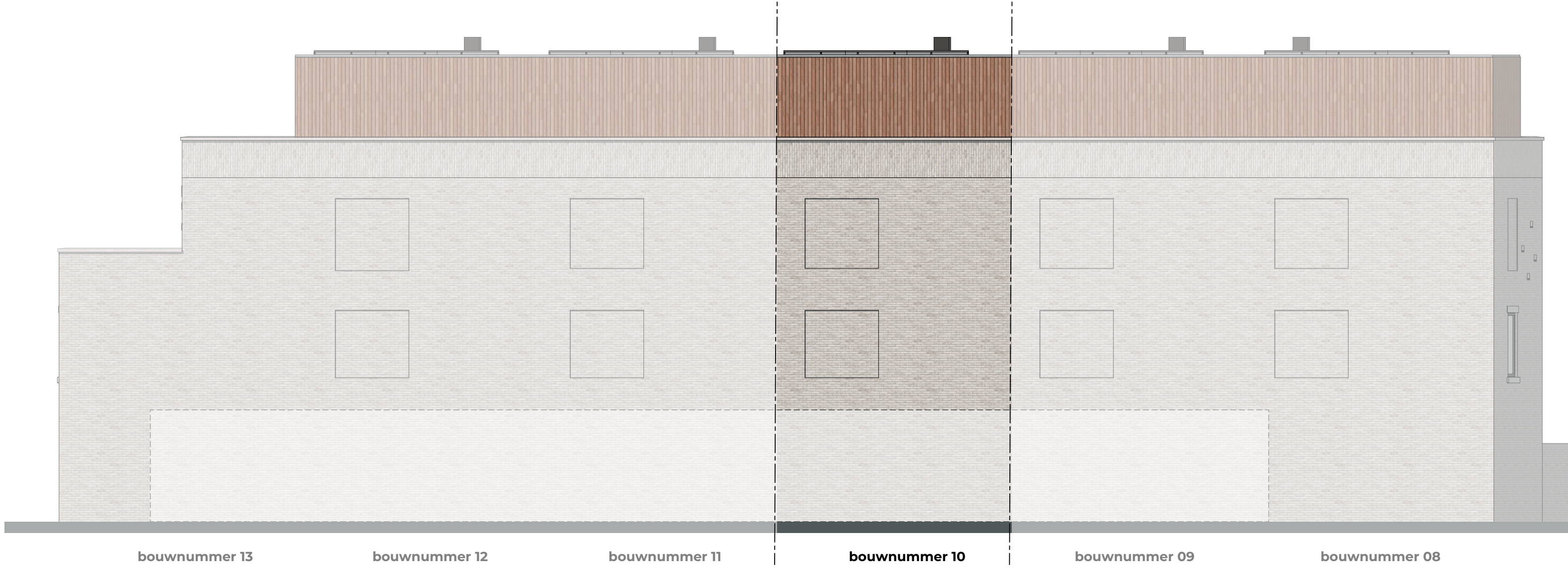
achtergevel schaal 1:100
