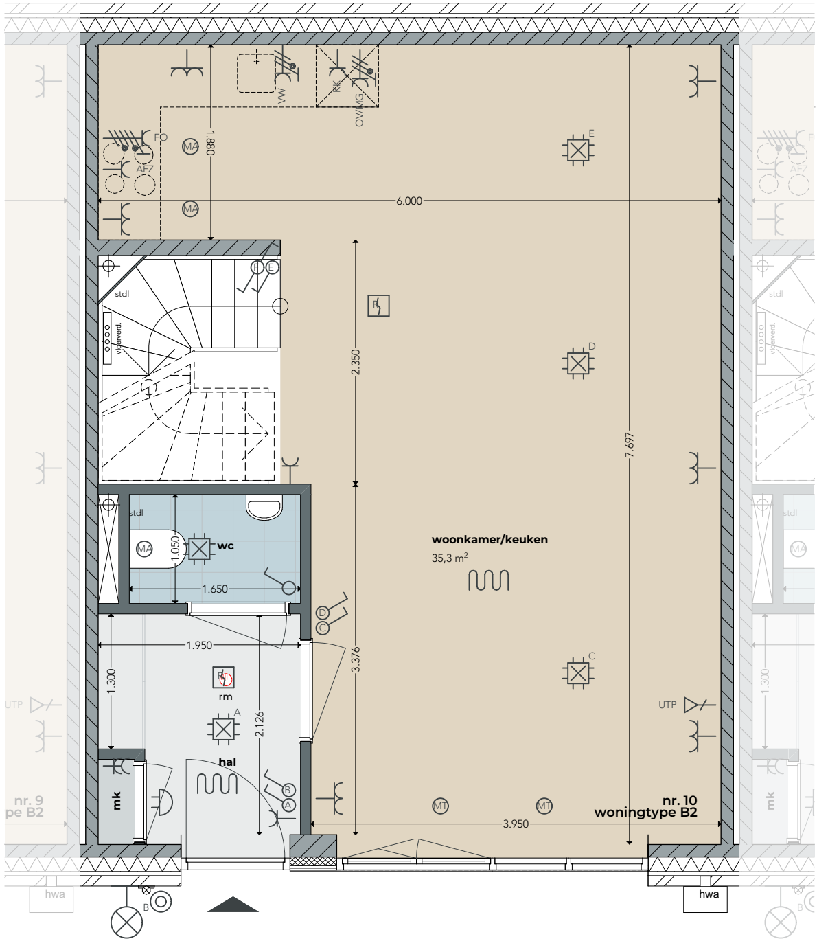
Begane grond schaal 1:50
