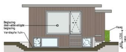
Doorsnede terrein bij linkerzijgevel woning 2.
